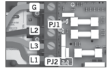
3 connexion en triangle de phase
