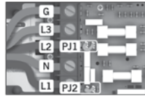
3 connexion de phase
